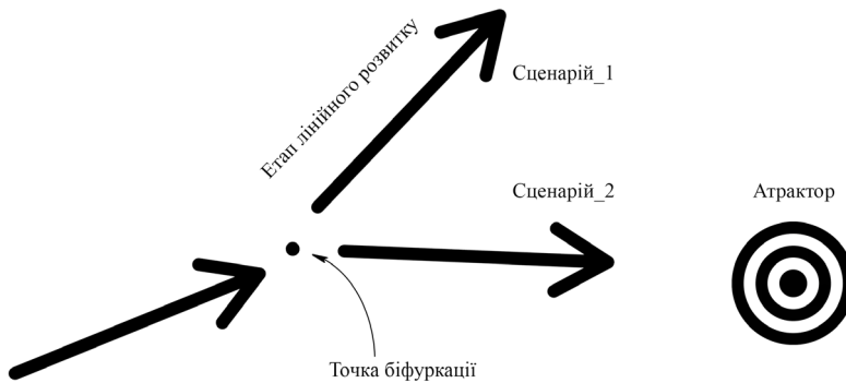
Рис. 1. Схема проходження точки біфуркації
